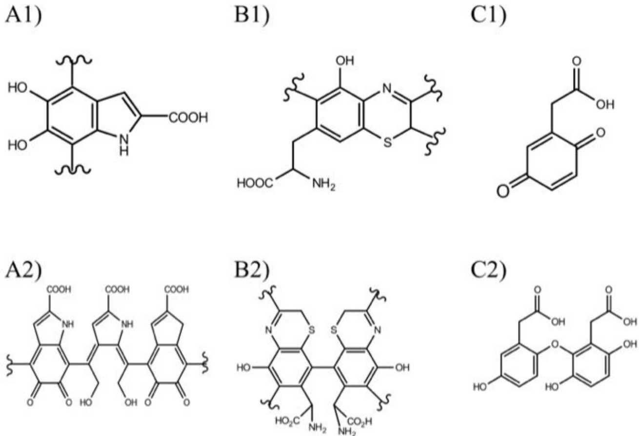
Figura 2. Monómeros (1) y polímeros (2) que forman las estructuras de diferentes tipos de melaninas: A) eumelanina, B) feomelanina, C) piomelanina y D) neuromelanina (autoría propia).
